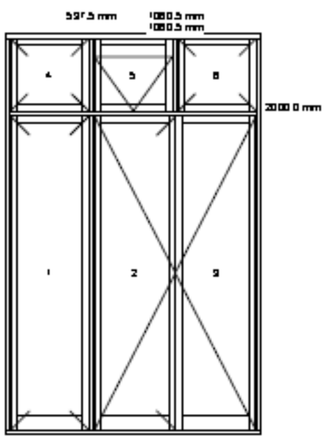
Døre altan type: 4 + 5
